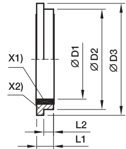
X1) Joint NBR X2) Bague de retenue (Acier)
